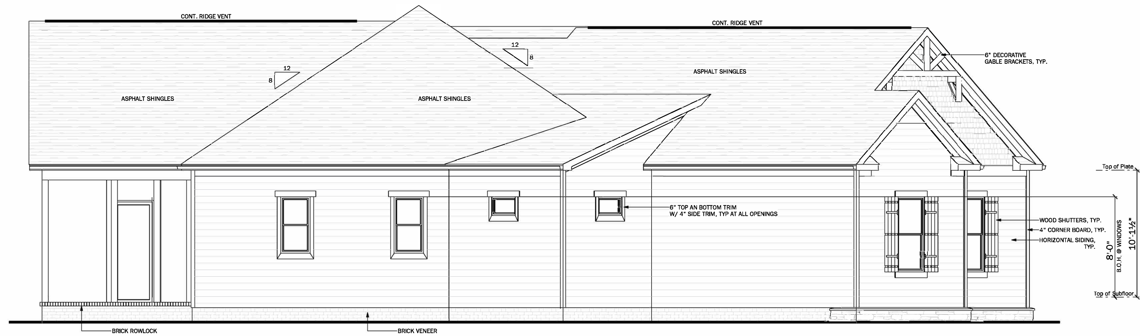
LEFT SCALE: 1/4" = 1'-0"
