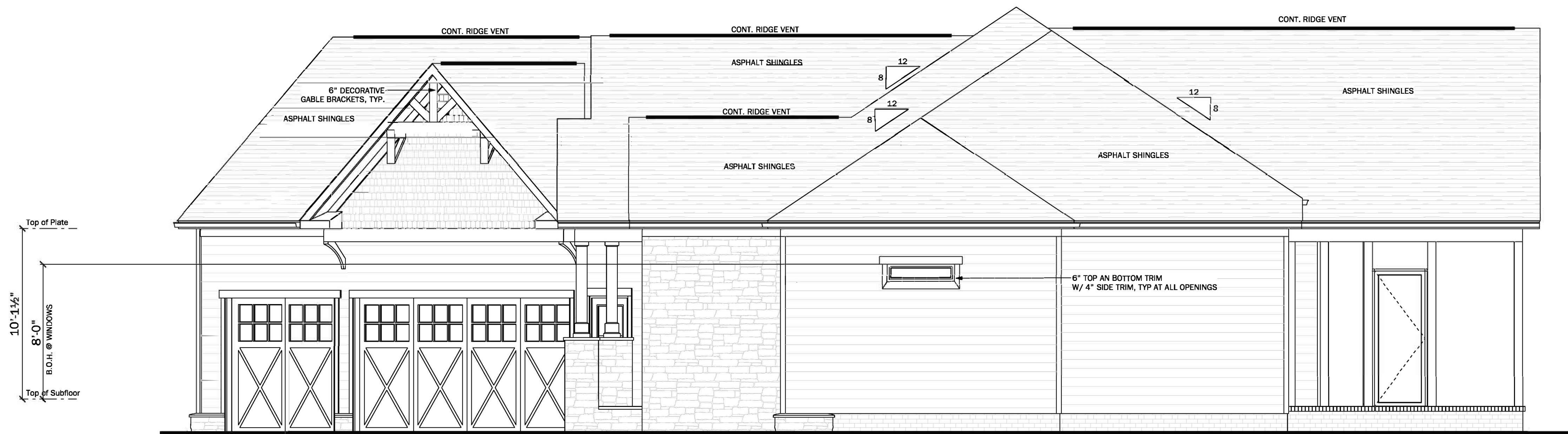
RIGHT SCALE: 1/4" = 1'-0"
