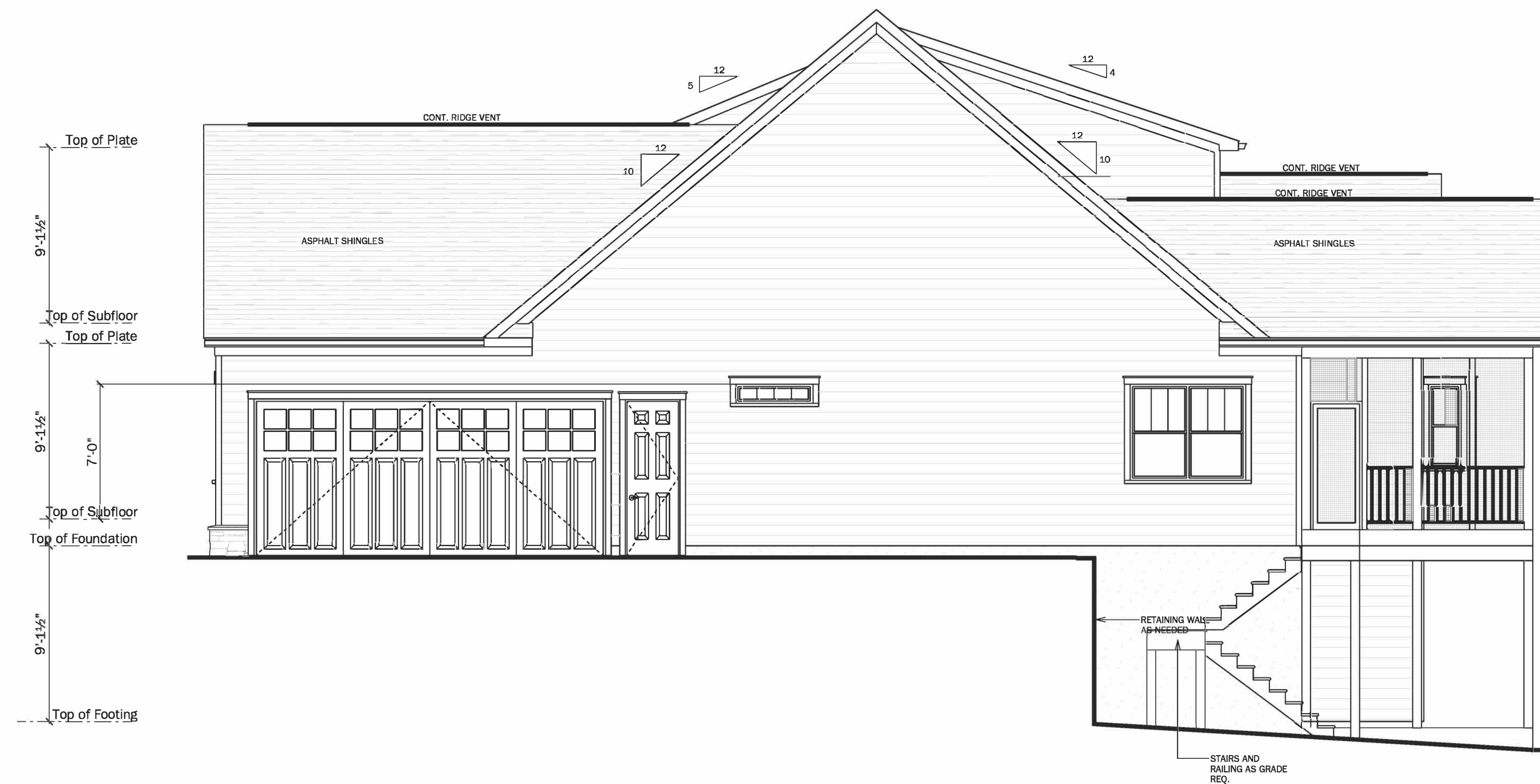
REAR SCALE: 1/4" = 1'-0"
