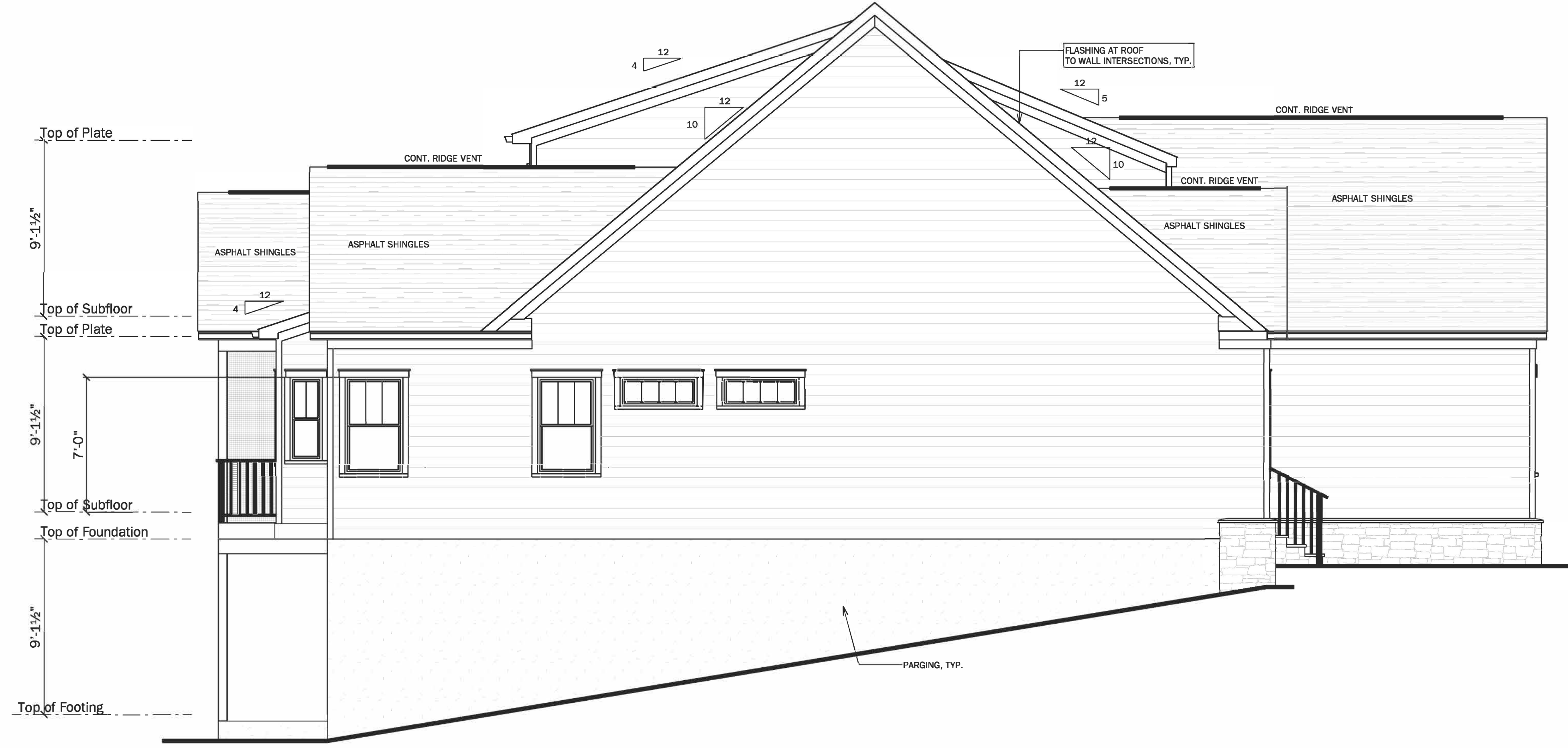
LEFT SCALE: 1/4" = 1'-0"
